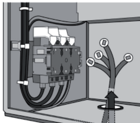
Otvor na spodku spínacej skrinky a svorkovnica pre elektrický prívod
