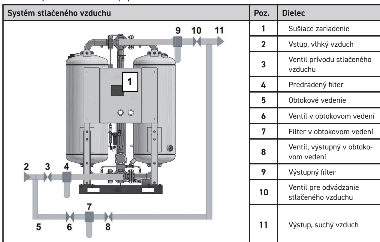
Príklad inštalácie s obtokovým vedením
