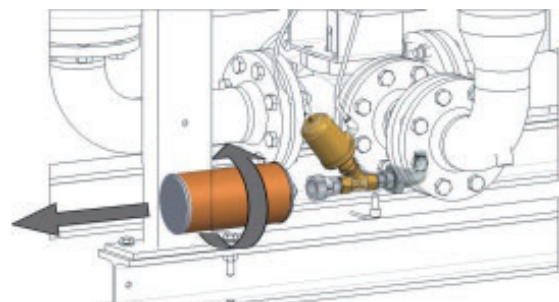
Uvoľnenie tlmiča hluku
