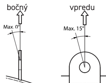
Preprava žeriavom
